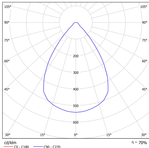
POLAR-KOORDINATEN DIAGRAMM
