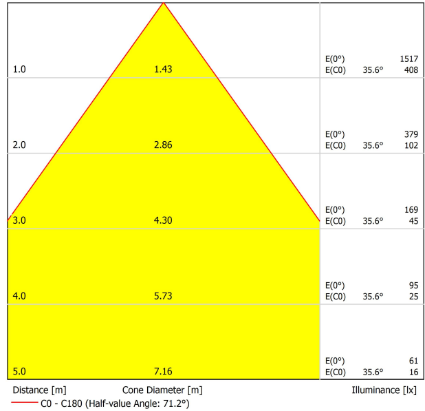
DIAGRAMMA CONICO
