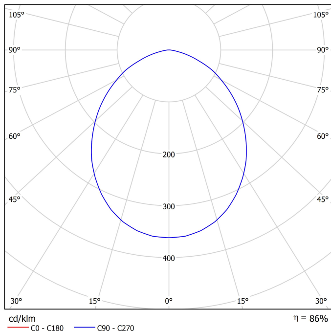
Diagrama cónico
