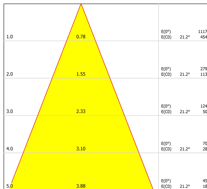
Diagramme conique
