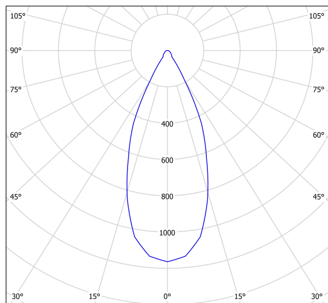
Diagramme polaire
