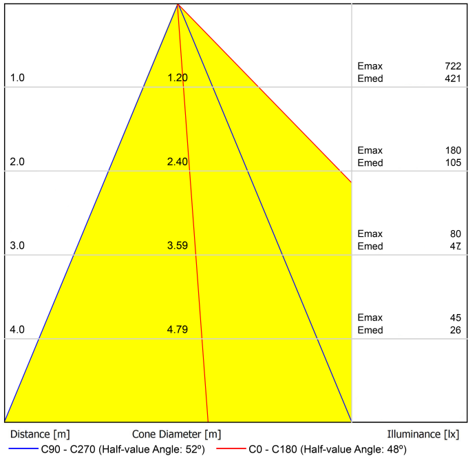
Diagrama cónico
