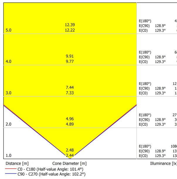
DIAGRAMME CONIQUE
