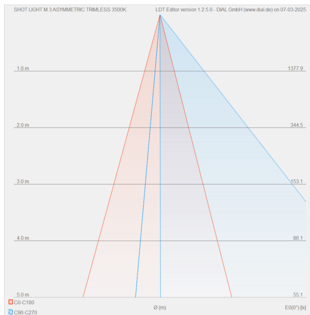
DIAGRAMA CÓNICO
