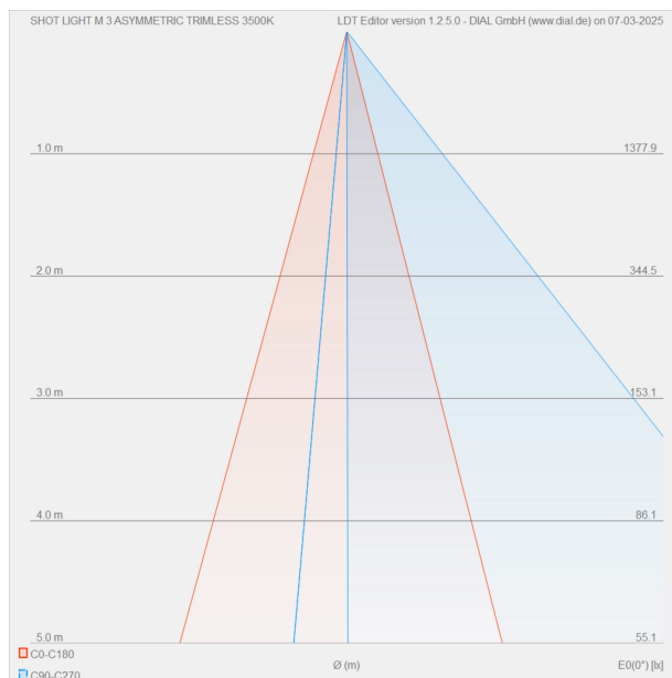
DIAGRAMA CÓNICO
