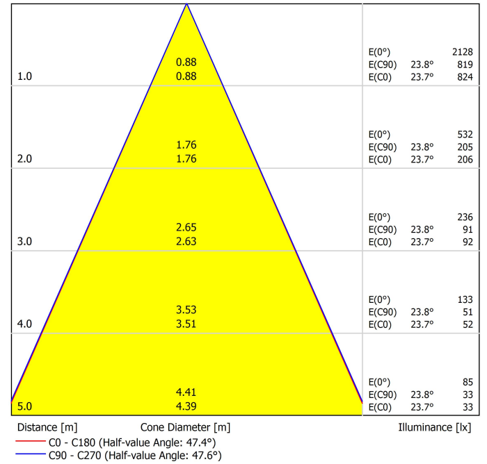
Diagrama cónico
