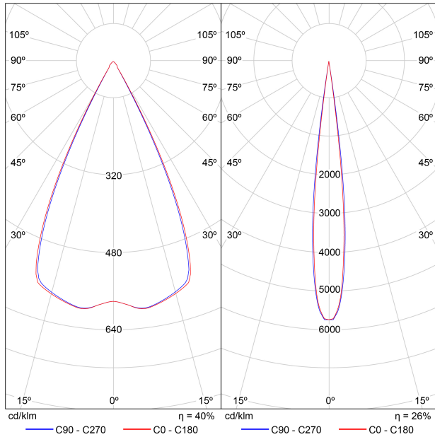
DIAGRAMME POLAIRE
