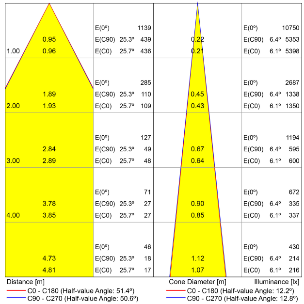
DIAGRAMME CONIQUE
