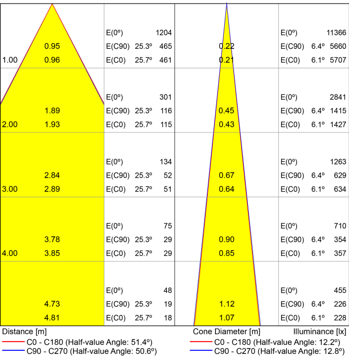
KEGELDIAGRAMM
