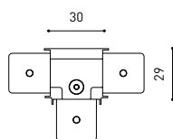
T-Joint
