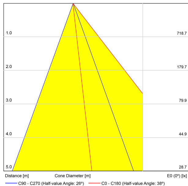
DIAGRAMMA CONICO
