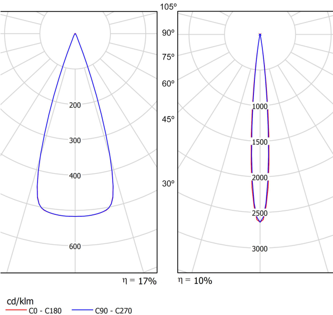
Diagramme polaire
