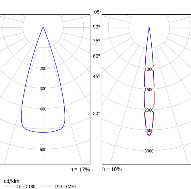
Diagramme polaire
