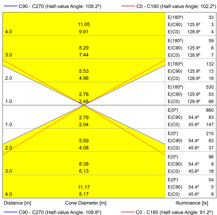
Diagrama cónico
