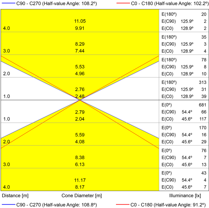
Diagramma conico
