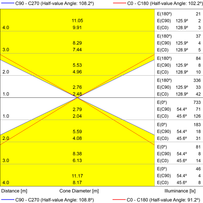
Kegeldiagramm
