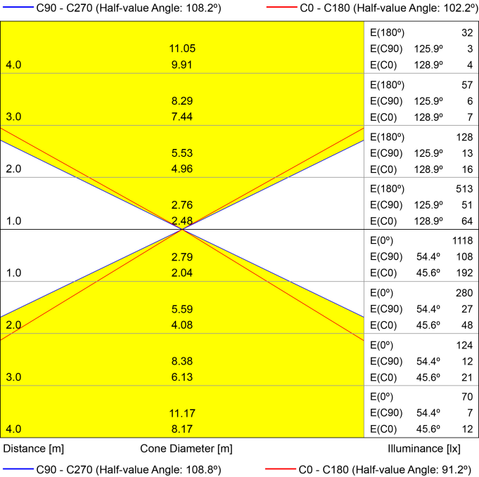
Diagrama cónico
