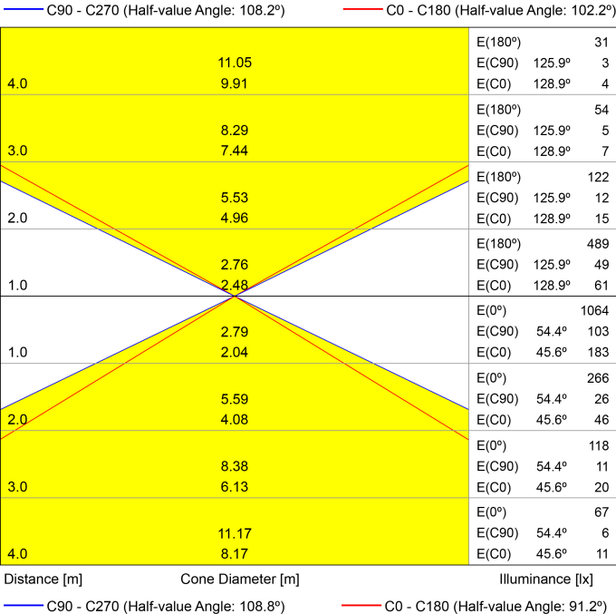
Diagrama cónico
