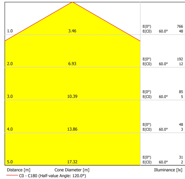
DIAGRAMMA CONICO
