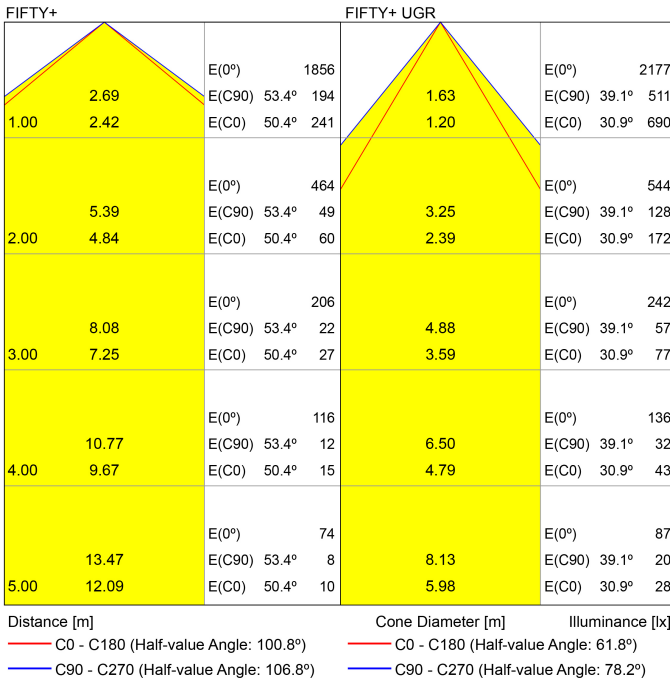
Diagrama cónico
