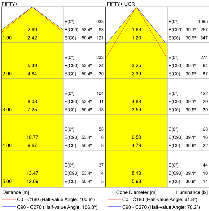
Diagrama cónico
