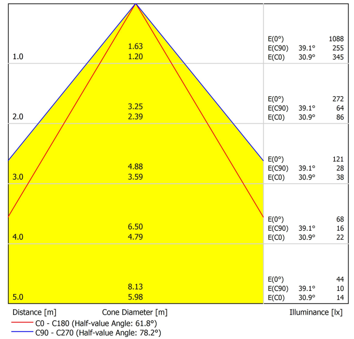
Diagrama cónico
