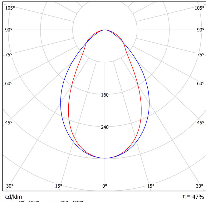
Diagrama polar
