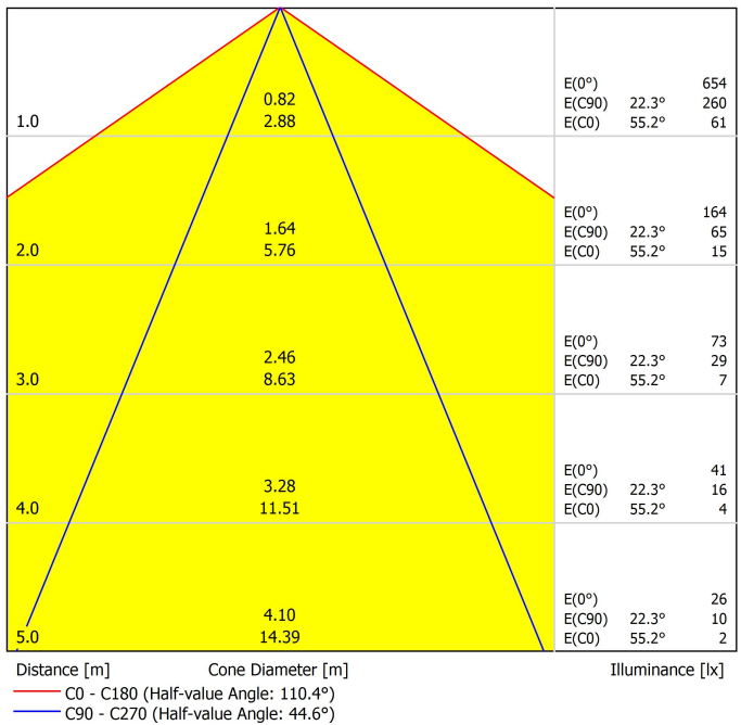
Kegeldiagramm
