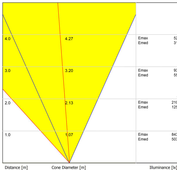
DIAGRAMA CÓNICO
