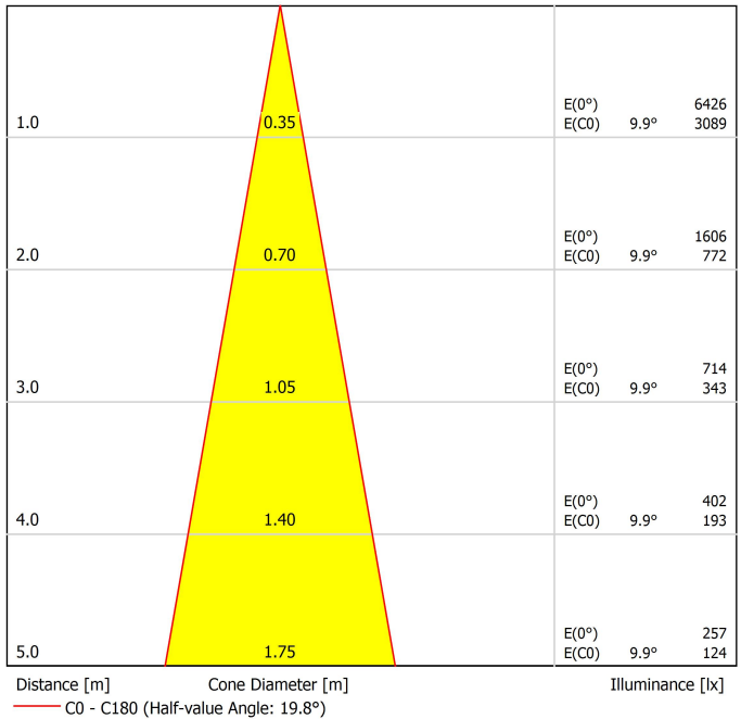
Kegeldiagramm
