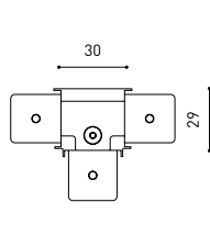
T-Joint
