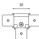
T-Joint
