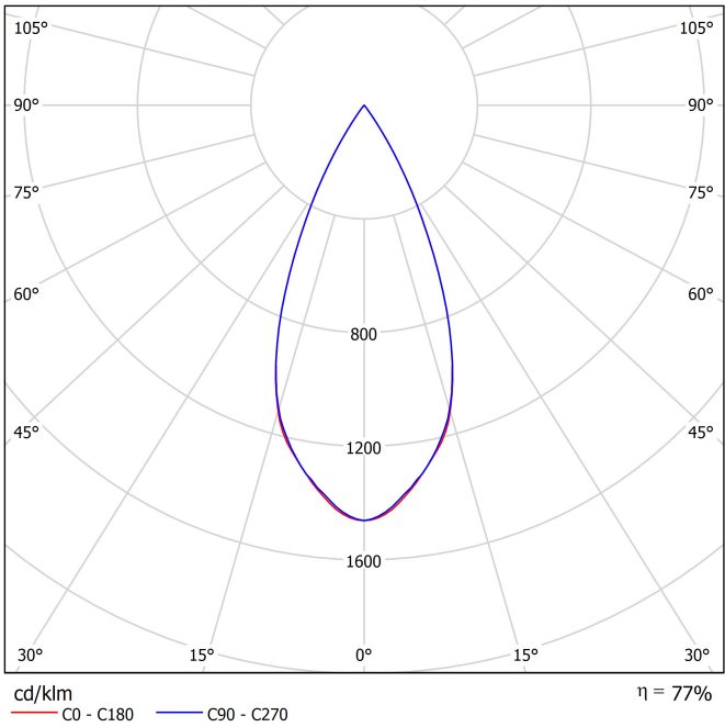
DIAGRAMMA DI ABBACLIAMENTO POLARE
