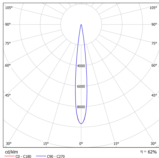
Diagrama polar
