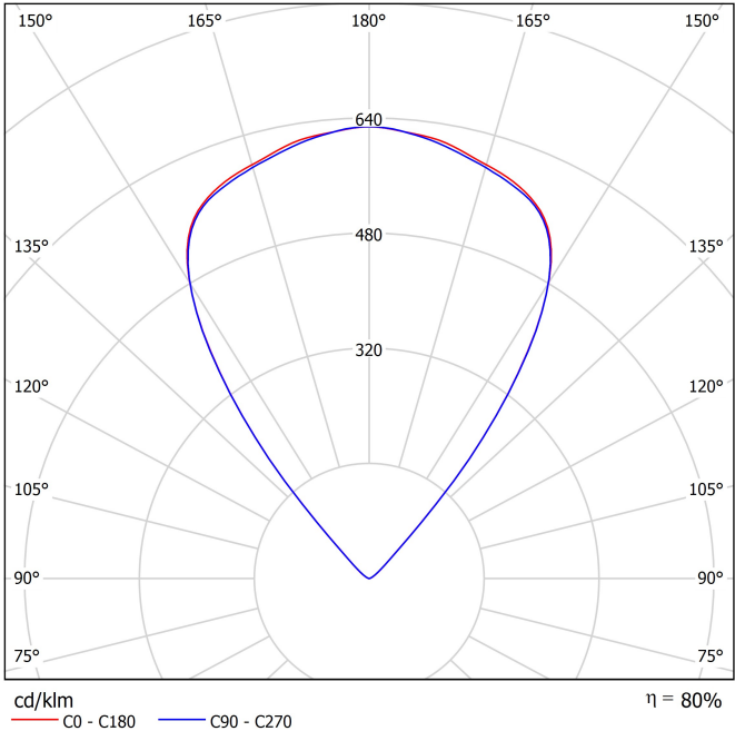
Diagrama polar
