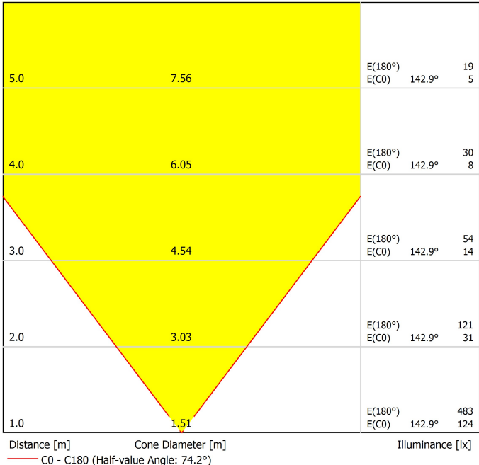
Diagrama cónico
